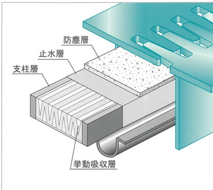
プレスアドラー構成図
