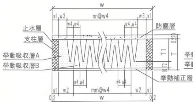
各遊間別断面寸法一覧表
