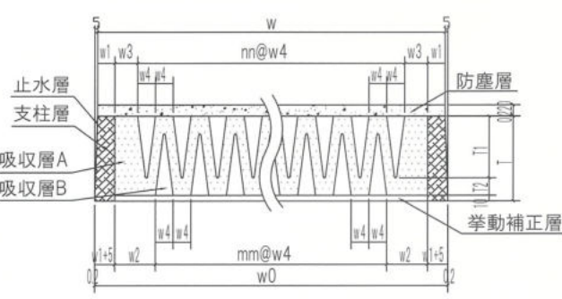
Type-200~700の場合の支柱層の寸法
